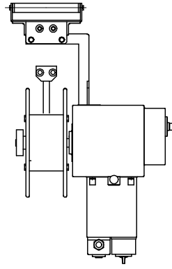
左仕様機
